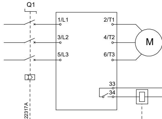
Softstarter mit Nebenschlussrelais und Schutzschalter
