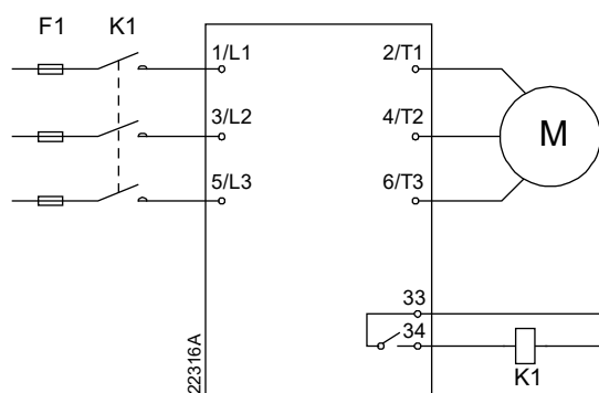
Softstarter mit Hauptschütz
