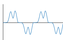
Standard-Frequenzumrichter
