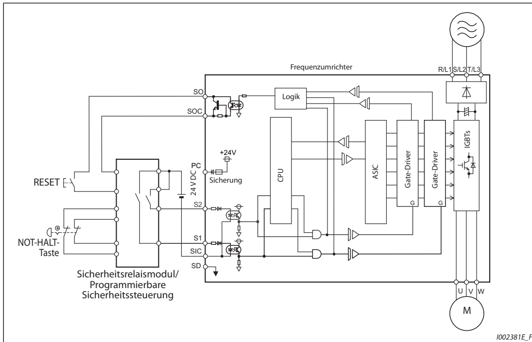
Abb. 2-44: Anschluss des Sicherheitsrelaismoduls
