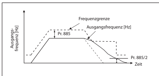
Abb. 5-364: Beschränkung der Ausgangsfrequenz
