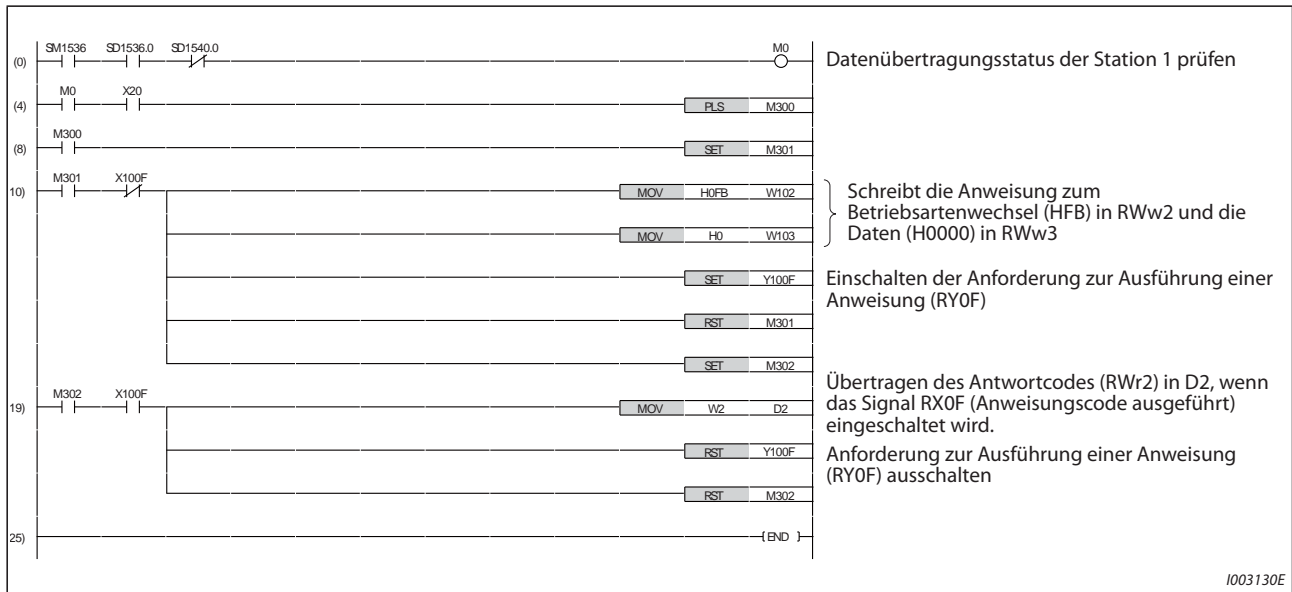
Abb. 5-395: Programmbeispiel 2
