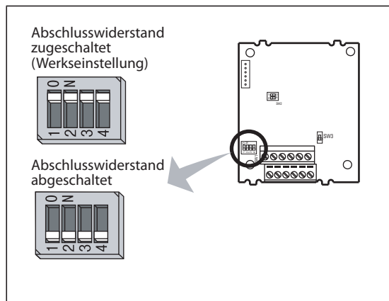
Abb. 2-50: Schalter zum Zuschalten des Abschlusswiderstandes
