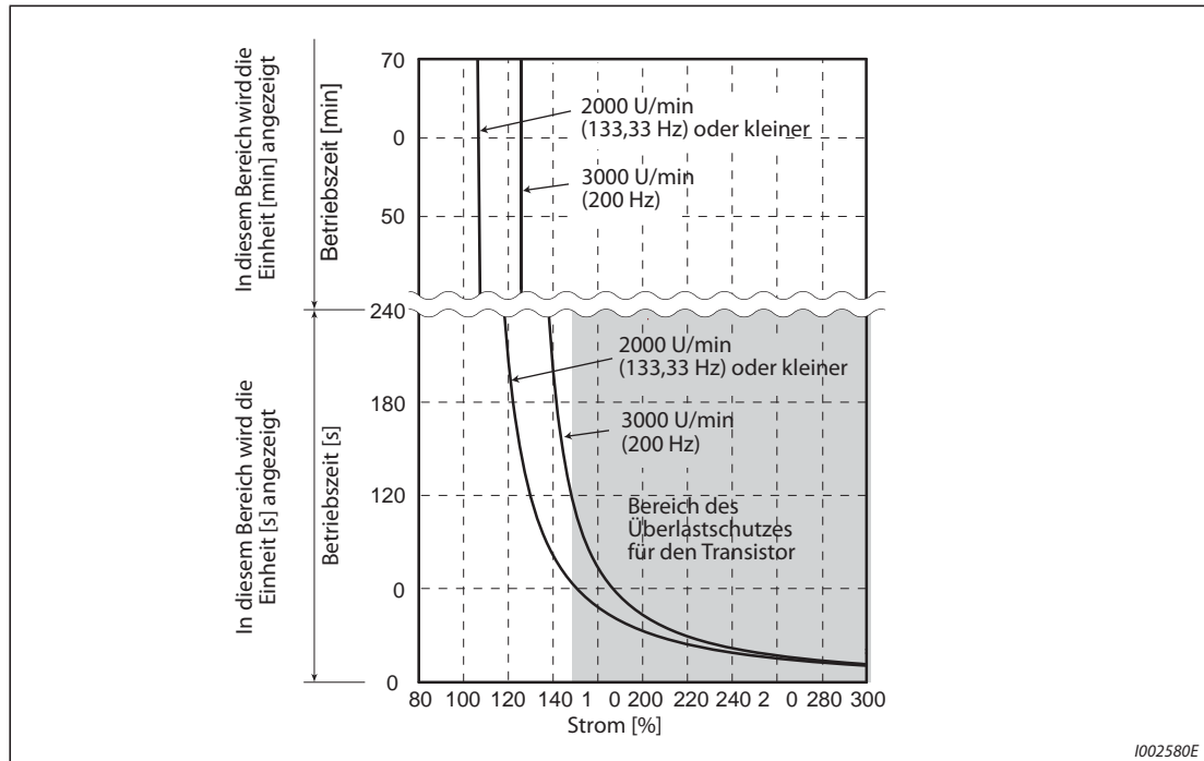
Abb. 5-123: Motorschutz-Kennlinien (MM-CF)
