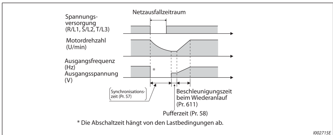
Abb. 5-291: Frequenzerfassung über Impulsgeber (Pr. 162 = 2/12)
