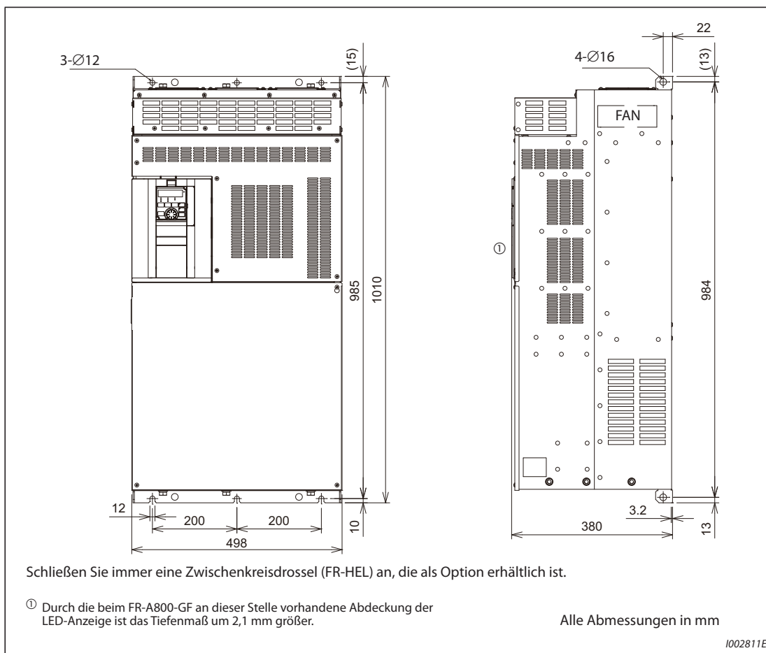
Abb. 8-7: Abmessungen der Frequenzumrichter FR-A840-04320(160K), 04810(185K)
