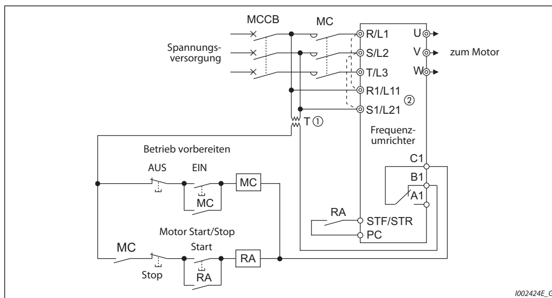
Abb. 3-12: Starten/Stoppen des Frequenzumrichters
