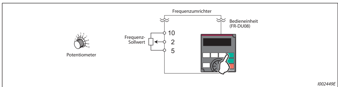
Abb. 5-113: Kombinierte Betriebsart 2
