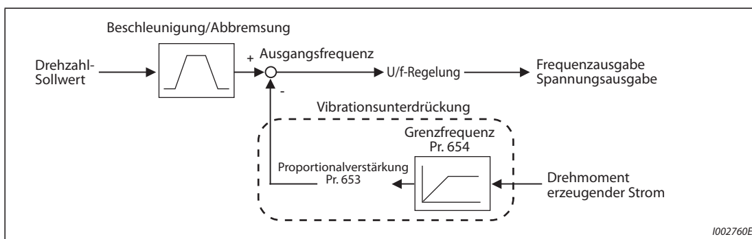
Abb. 5-368: Blockschaltbild
