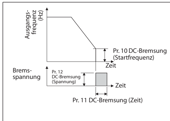
Abb. 5-347: Einstellung des Pr. 11 auf einen Wert zwischen 0,1 und 10 s
