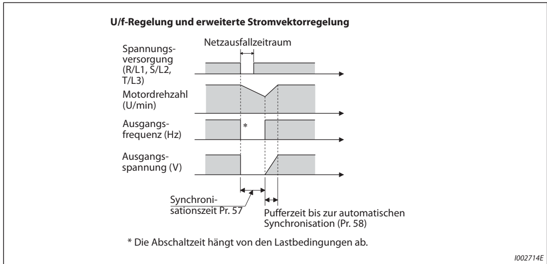
Abb. 5-290: Automatischer Wiederanlauf ohne Ausgangsfrequenzerfassung (Pr. 162 = 1/11)
