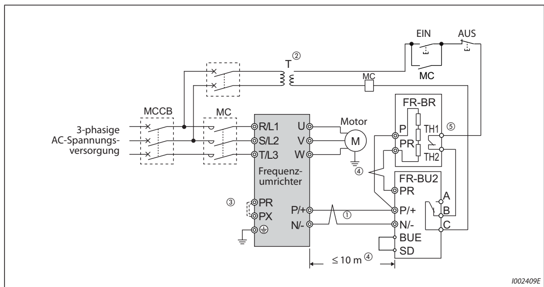
Abb. 2-64: Anschluss der Bremseinheit mit dem Bremswiderstand FR-BR(-H)
