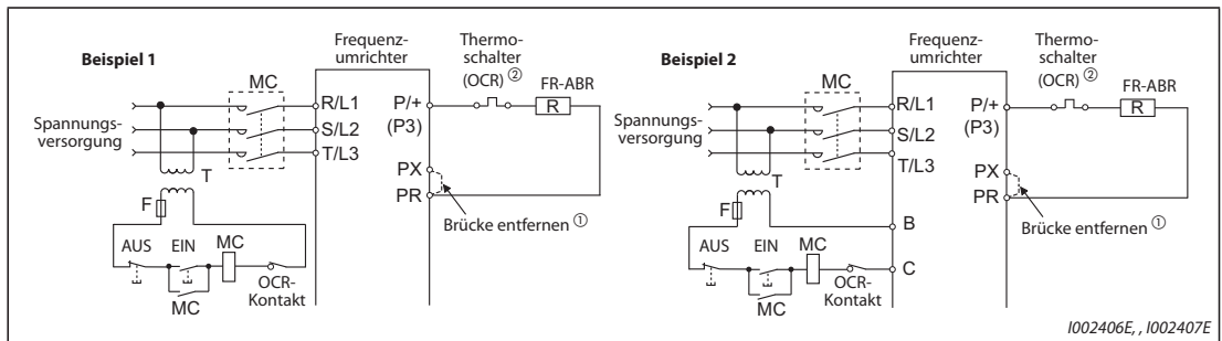
Abb. 2-61: Schutzschaltung
