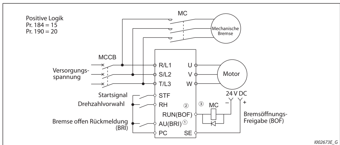
Abb. 5-234: Anschlussbeispiel mit mechanischer Bremse (Pr. 184 = 15, Pr. 190 = 20)
