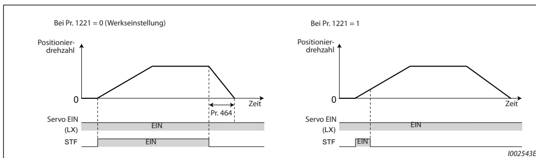
Abb. 5-64: Abrupter Stopp
