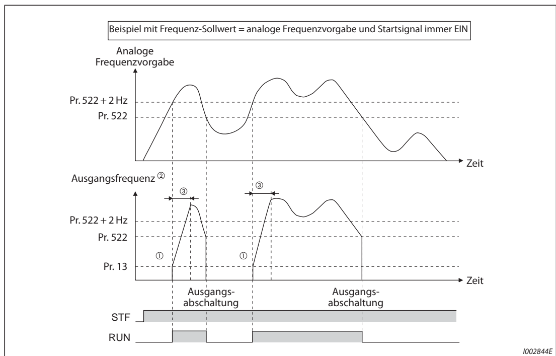
Abb. 5-353: Beispiel für die Ausgangsabschaltung
