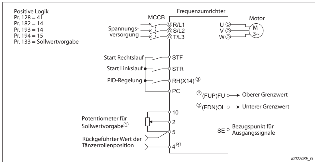
Abb. 5-282: Anschlussbeispiel in positiver Logik
