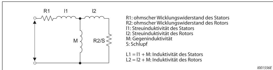
Abb. 5-222: Motorersatzschaltbild
