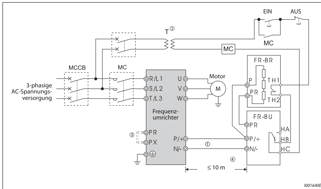
Abb. 2-66: Anschluss der Bremsseinheit FR-BU
