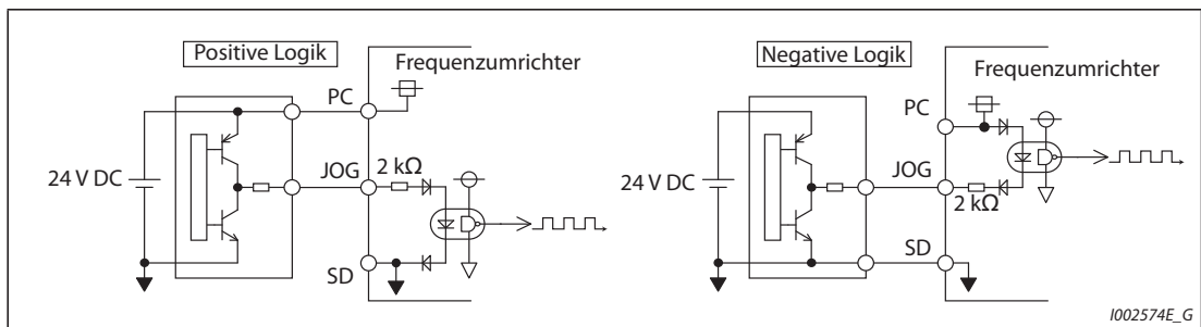
Abb. 5-115: Impulsausgang
