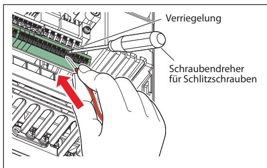
Abb. 2-34: Anschluss einer verlitzen Leitung
