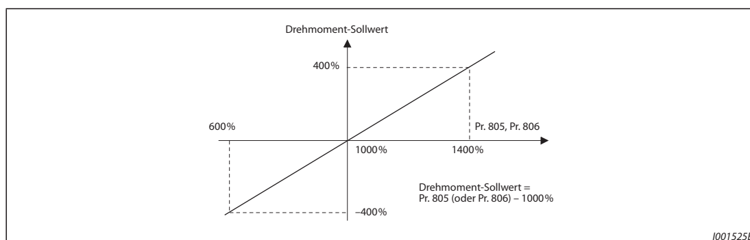
Abb. 5-46: Vorgabe des Drehmoment-Sollwerts über Parameter
