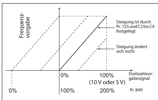
Abb. 5-203: Offset-Einstellung
