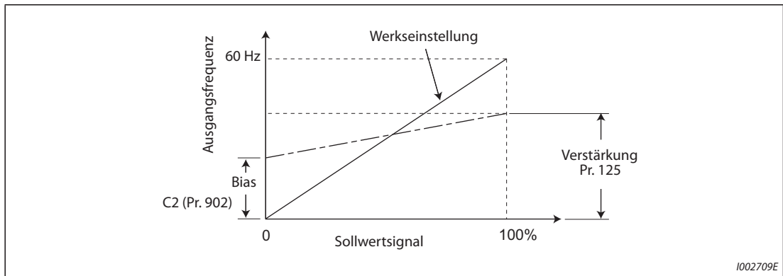
Abb. 5-283: Signalabgleich an Klemme 2
