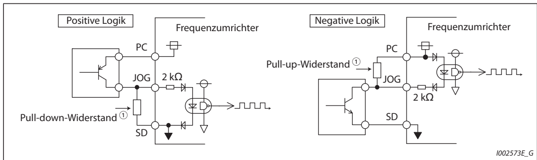
Abb. 5-114: Impulseingang
