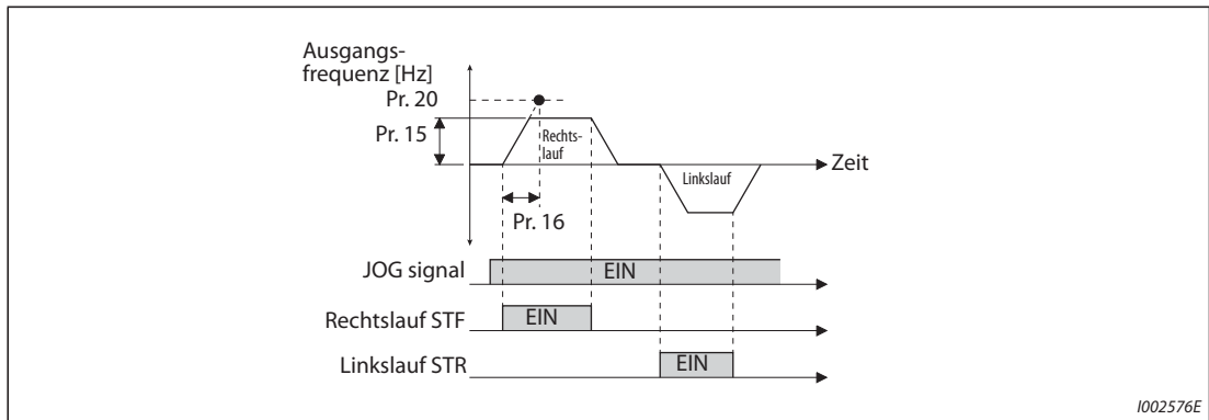
Abb. 5-118: Zeitverläufe der Signale im Tippbetrieb
