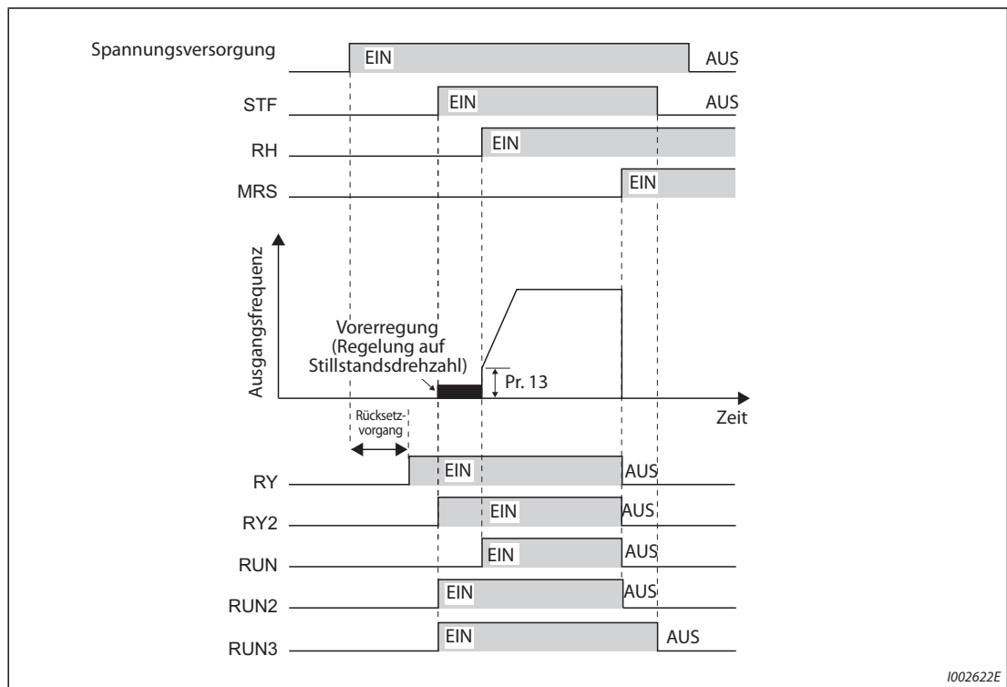
Abb. 5-171: Betriebsbereitschaft und Motorlauf
