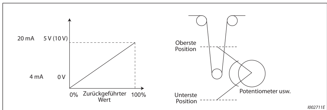
Abb. 5-285: Abgleich des Signals zur Positionserfassung der Tänzerrolle
