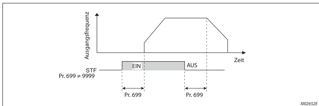
Abb. 5-213: Wirkungsweise der Ansprechverzögerung der Eingangsklemmen (Pr. 699)
