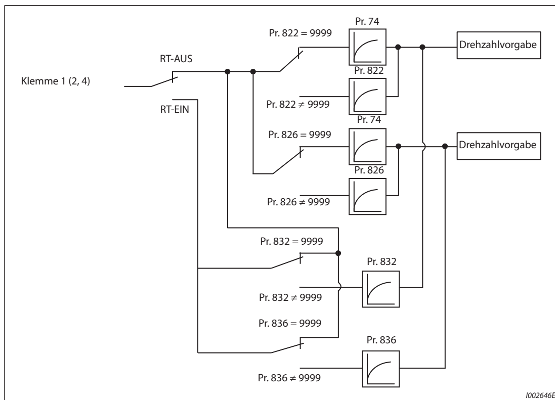
Abb. 5-202: Blockdiagramm der Eingangsklemme 1 (2, 4)
