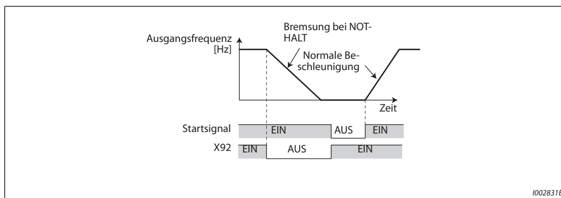
Abb. 5-89: Beschleunigung und Abbremsung bei aktivierter NOT-HALT-Funktion
