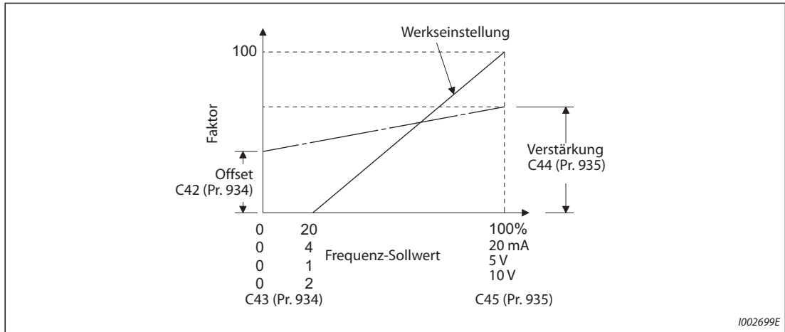
Abb. 5-274: Offset und Verstärkung für PID-Anzeigewerte
