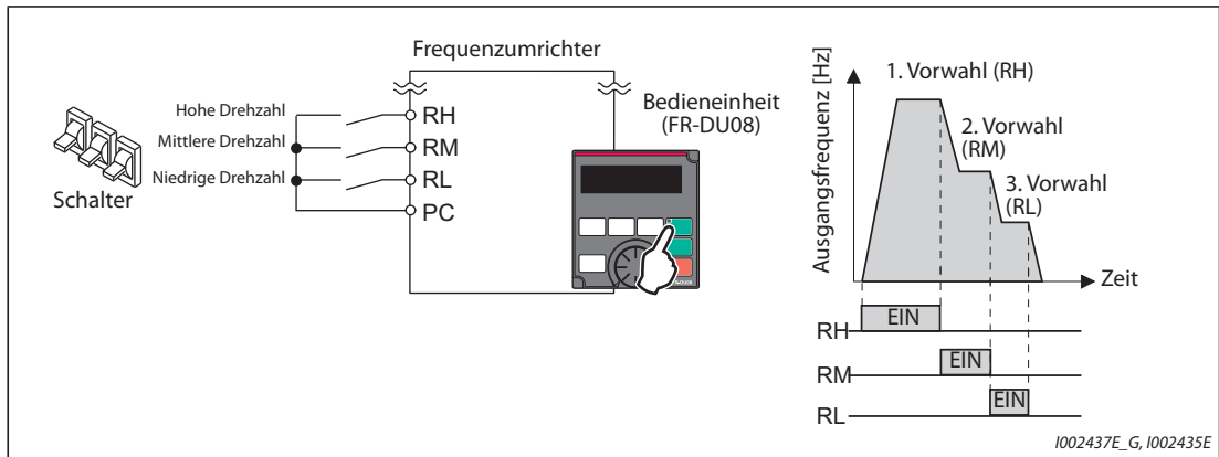
Abb. 4-5: Drehzahl-/Geschwindigkeitsvorwahl über Schalter
