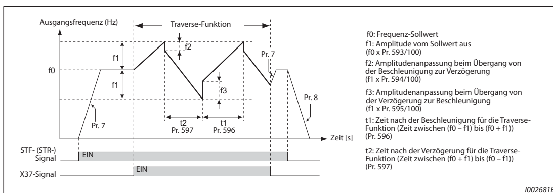
Abb. 5-245: Traverse-Funktion
