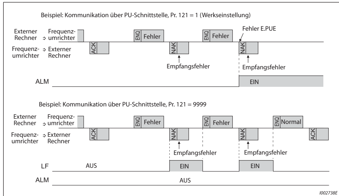
Abb. 5-322: Datenübertragungsfehler
