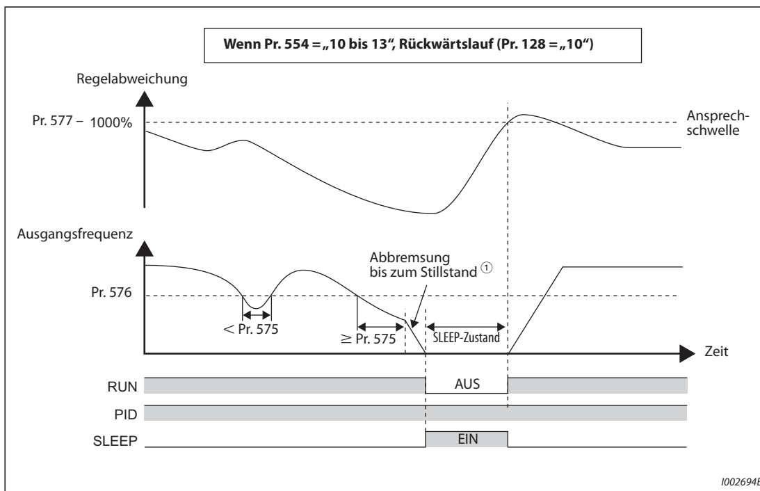
Abb. 5-271: Ausgangsabschaltung (SLEEP-Funktion)
