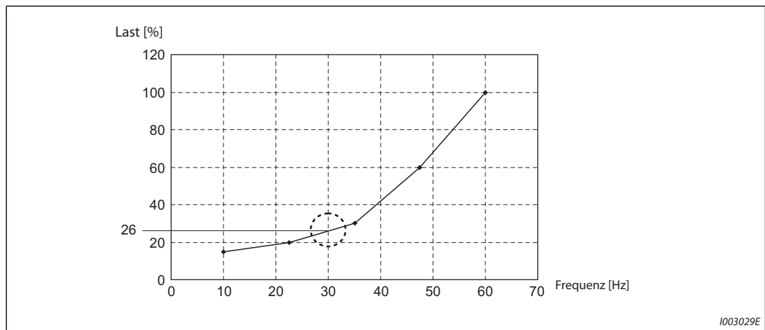
Abb. 5-149: Referenzwert bei einer Ausgangsfrequenz von 30 Hz
