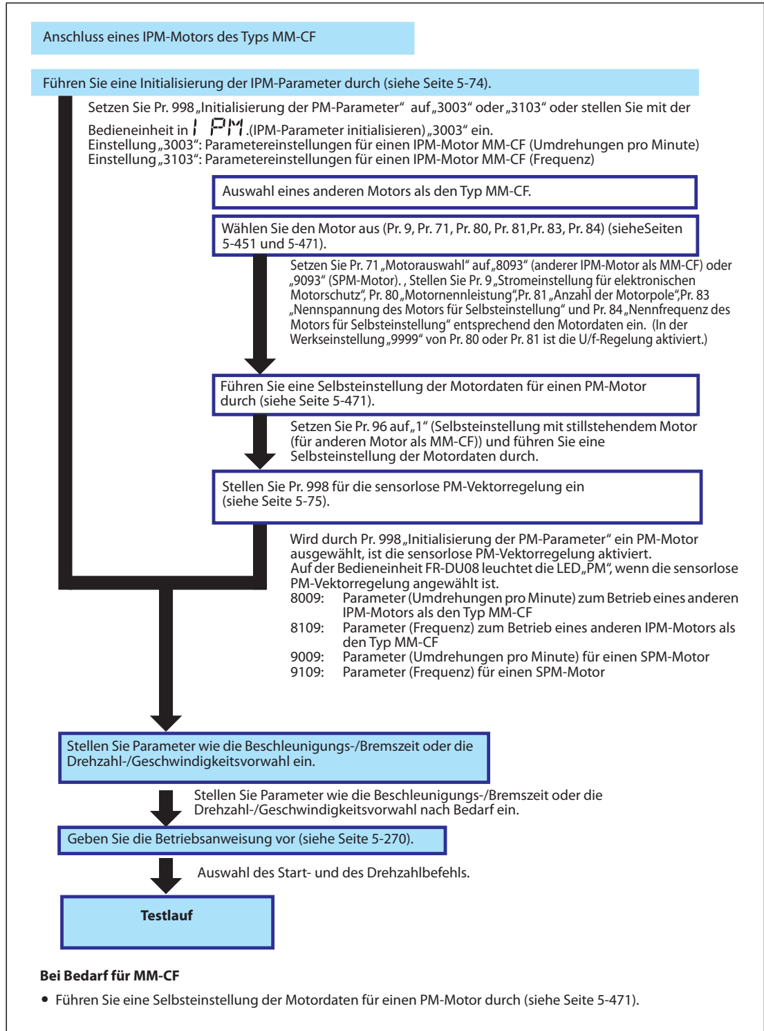
Abb. 5-12: Auswahlmethode der sensorlosen PM-Vektorregelung (Drehzahlregelung)
