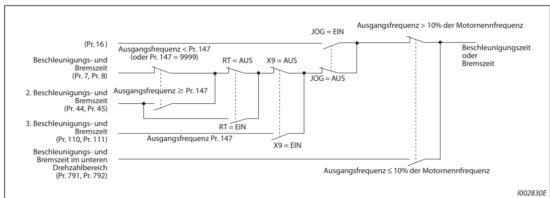
Abb. 5-85: Blockschaltbild
