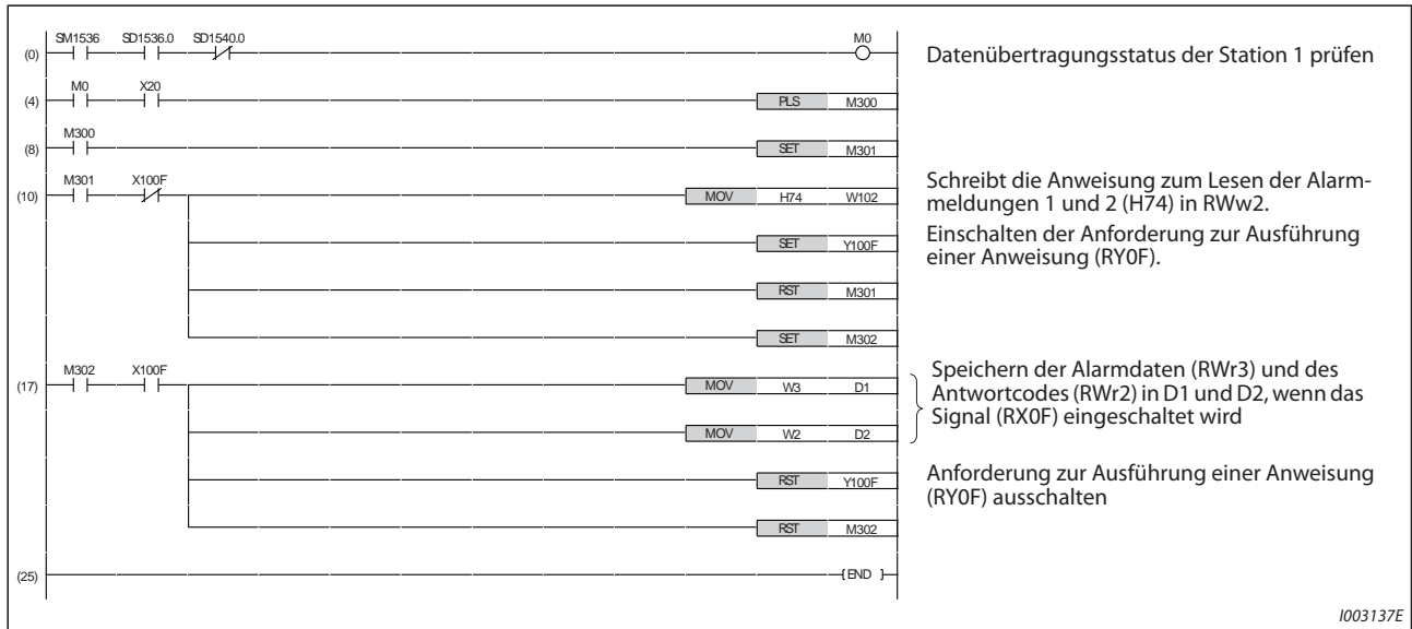
Abb. 5-400: Programmbeispiel 7
