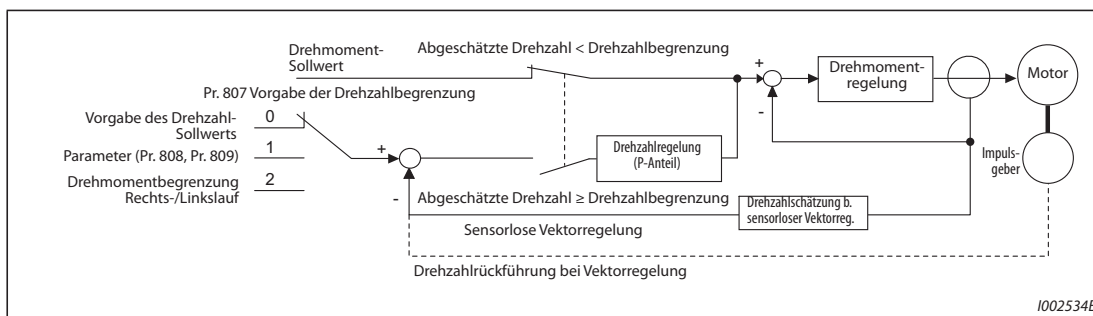
Abb. 5-48: Blockschaltbild
