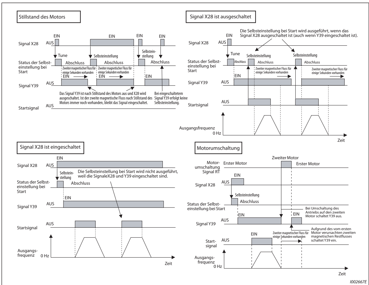
Abb. 5-224: Zeitdiagramme der Selbst-einstellung der Betriebsmotordaten
