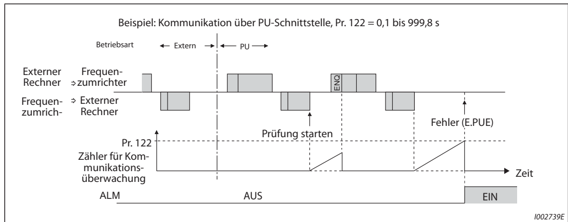
Abb. 5-323: Kabelbruchüberwachung
