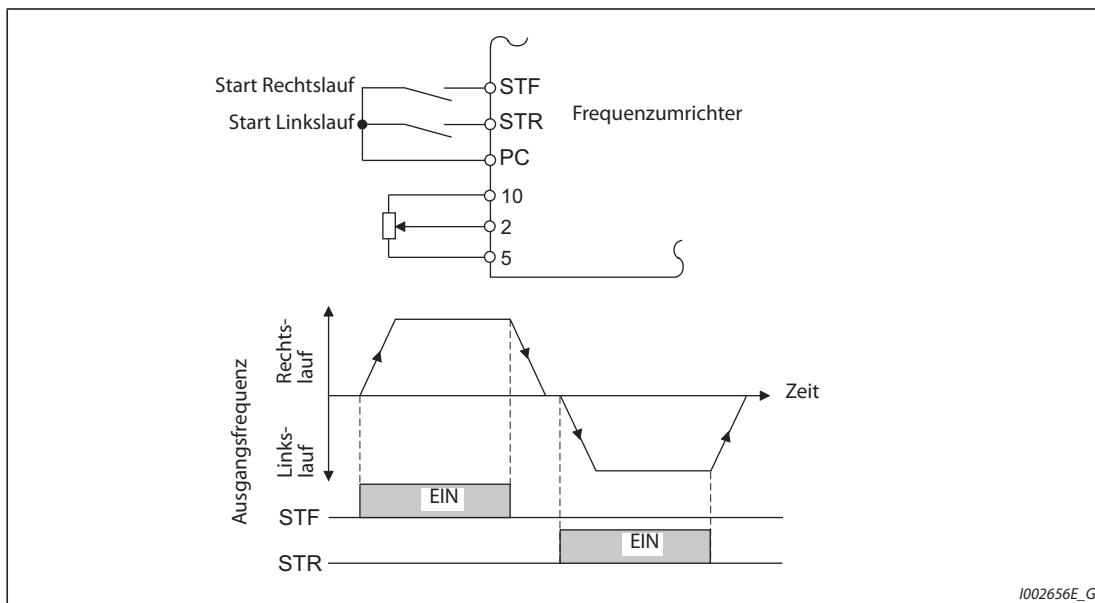
Abb. 5-218: Ansteuerung über eine 2-adrige Steuerleitung (Pr. 250 = 9999)
