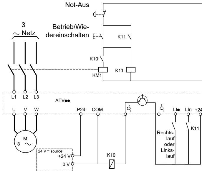
Spannungsversorgung 24 V
