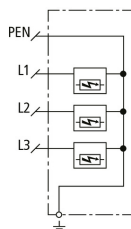
Prinzipschaltbild DSH ZP B2 TNC 255
