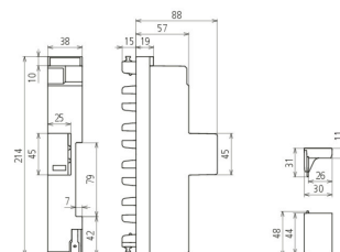
Maßbild DSH ZP B2 TNC 255
